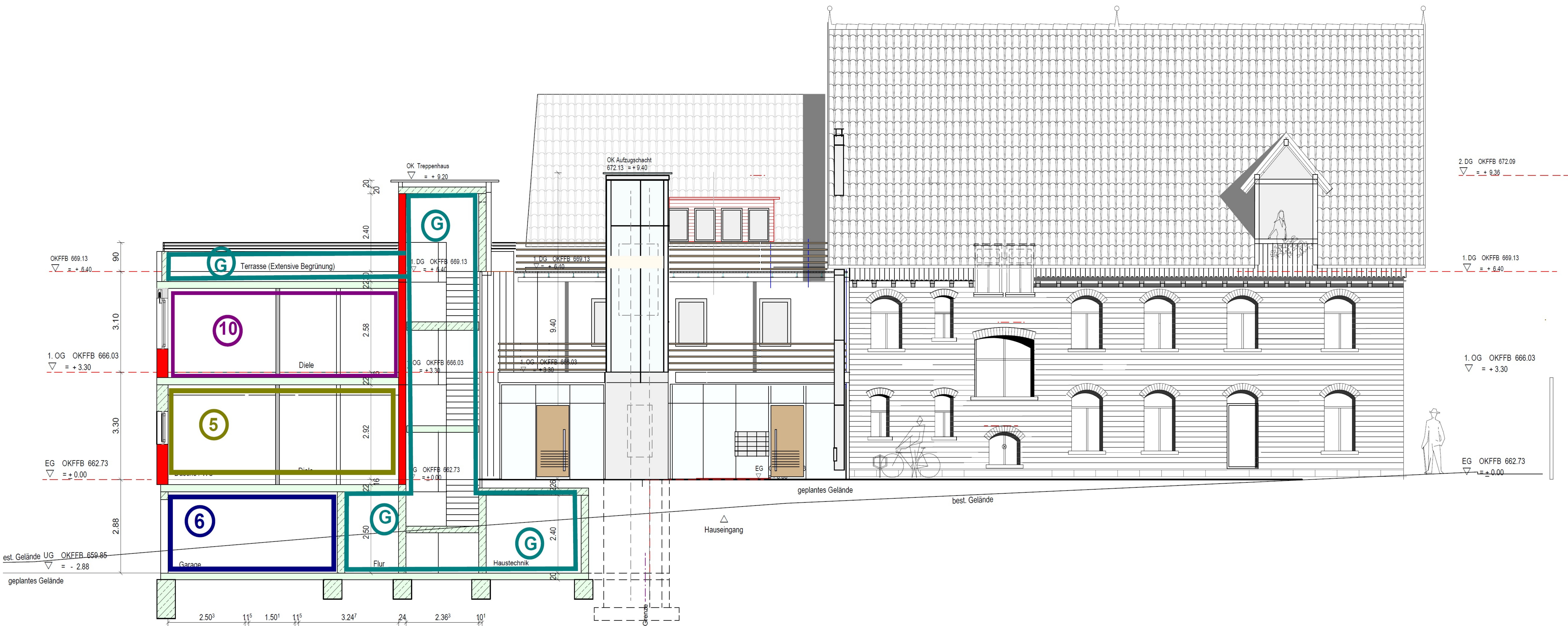
Ansicht Süd
